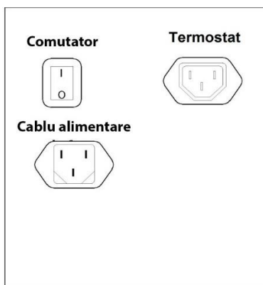
Figura 11: Conectarea termostatalui ambiental, direcționarea pompei (Buton PORNIT/OPRIT; Termostat; Cablu de alimentare)
