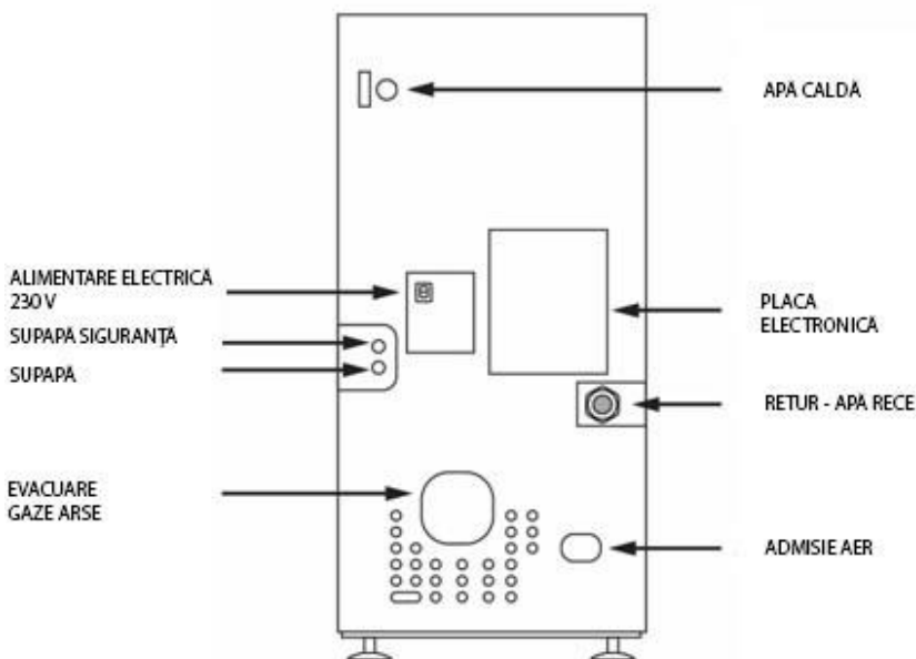
Figura 30. Pozitionarea racordurilor și a componentelor pe spatele termoșemineului
