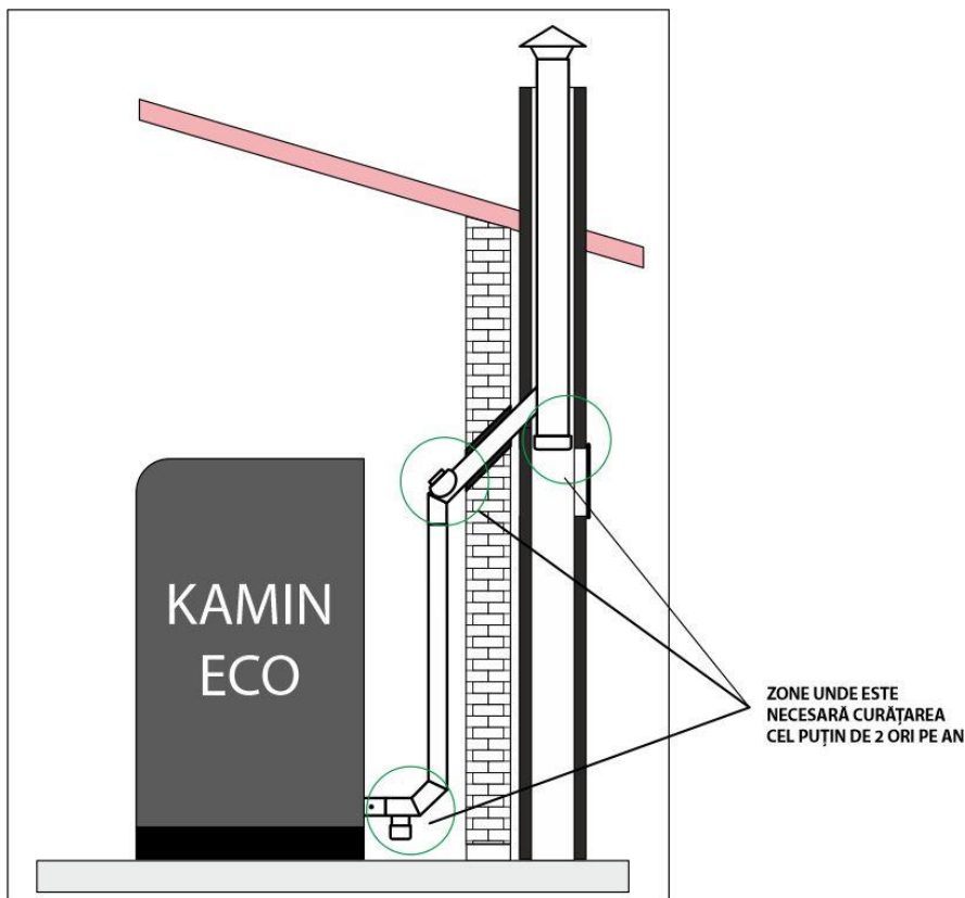
Figura 20. Zone care trebuie curățate cel puțin de două ori pe an.
