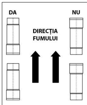
Figura 3. Montarea țevii pentru evacuarea fumului
