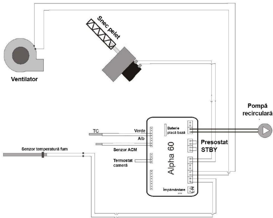
Figura 30: Schema electrică
