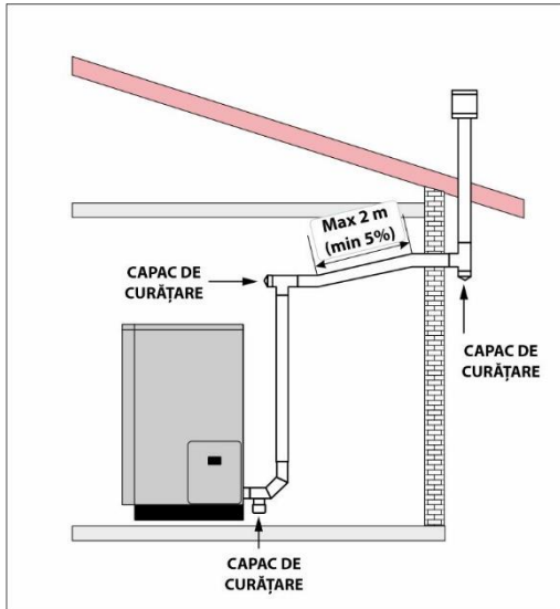
Figura 10. Panta minimă și lungimea maximă a sectoarelor orizontale
