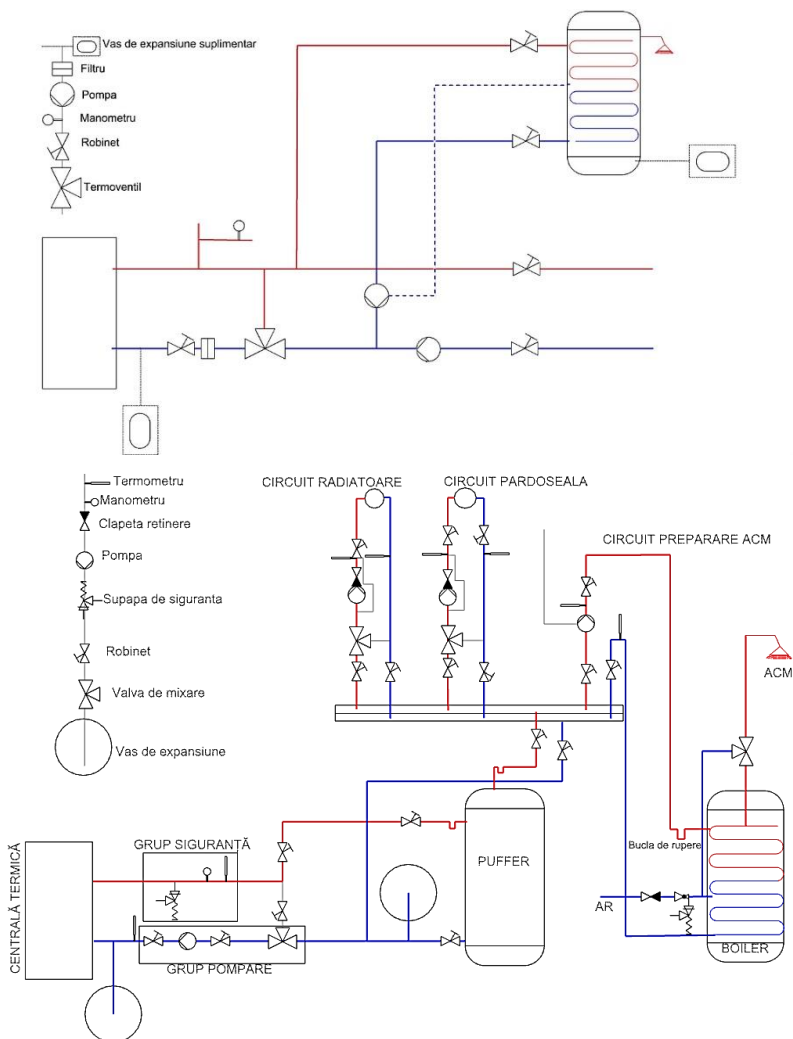
Figura 29. Schema instalației hidraulice
