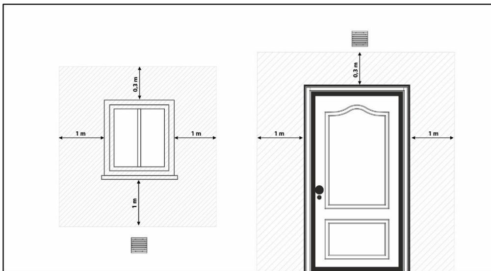
Figura 16. Distanțele minime pentru montarea grilei de ventilație
