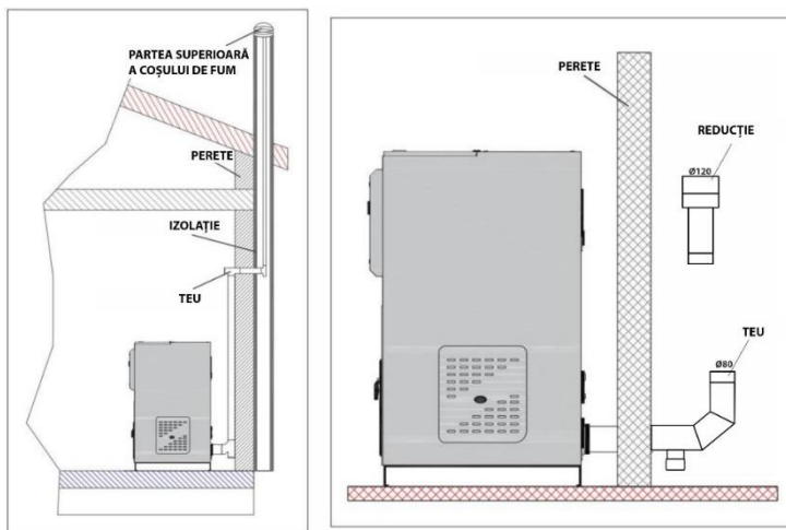
Figura 13. Grosimea și izolația țevii
